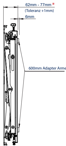
SEITENANSICHT GESCHLOSSEN
