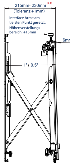
SEITENANSICHT VERLÄNGERT
