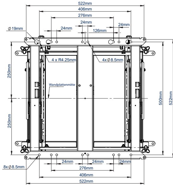
RÜCKANSICHT
