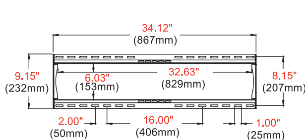
WANDPLATTE
