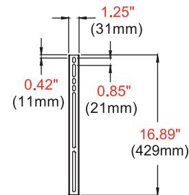
VERTIKALER ADAPTER
