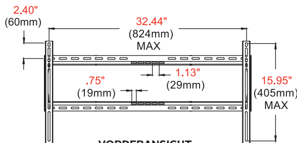
VORDERANSICHT
